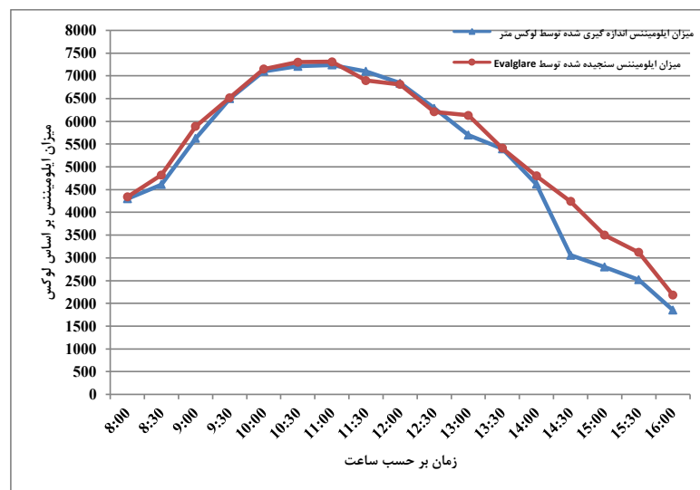
شکل ۹. مقایسه میزان روشنایی عمودی اندازه‌گیری شده توسط لوکس متر HS-1010 و سنجیده شده توسط Evalglare در ساعات متفاوت روز دوم مهرماه
