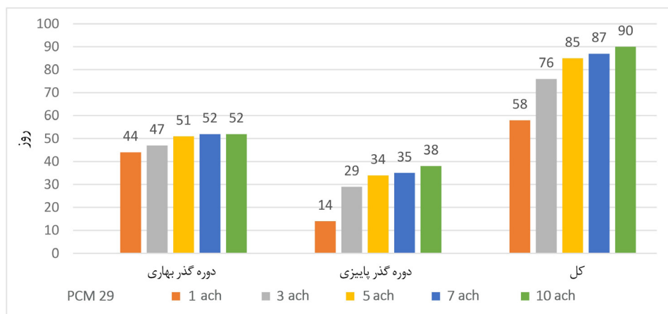
شکل ۲۱. میزان تأثیر تهویه طبیعی با نرخ تعویض هوای متفاوت بر افزایش تعداد روز دوره گذر فصلی در کل سال با میزان مصرف تا ۵ kWh / روزانه، با PCM 29
