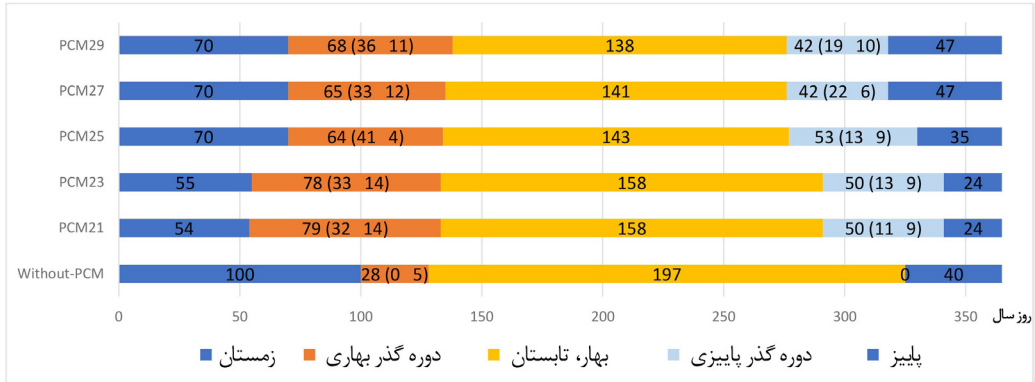
شکل ۲۴. طول و موقعیت دوره گذر فصلی در سال، تا ۵ kWh / روزانه مصرف انرژی، با نرخ تهویه ۳ ach
