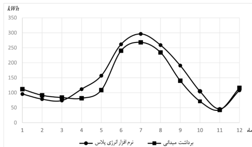
شکل ۳. برداشت میدانی و شبیه‌سازی نرم‌افزار انرژی پلاس
