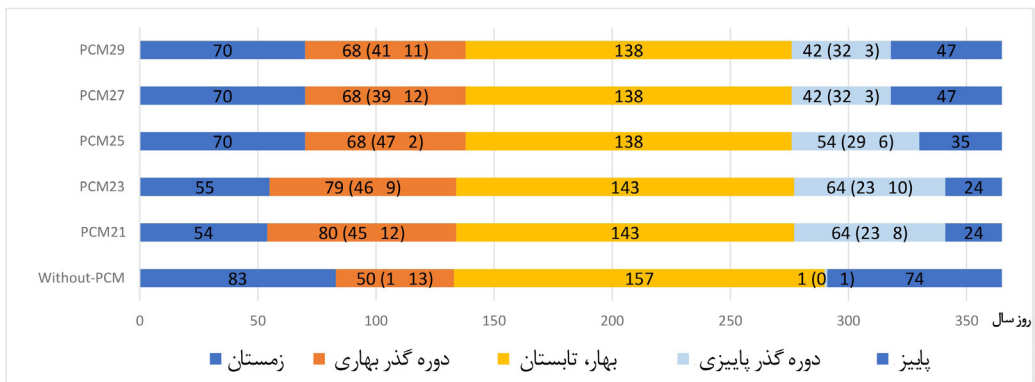
شکل ۲۶. طول و موقعیت دوره گذر فصلی در سال، تا ۵ kWh / روزانه مصرف انرژی، با نرخ تهویه ۷ ach
