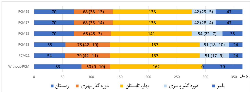
شکل ۲۵. طول و موقعیت دوره گذر فصلی در سال، تا ۵ kWh / روزانه مصرف انرژی، با نرخ تهویه ۷ ach
