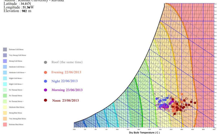
شکل ۸. نمودار UTCI در ۲ و ۳ تیر ۱۳۹۲ پردیس دانشگاه کاشان
