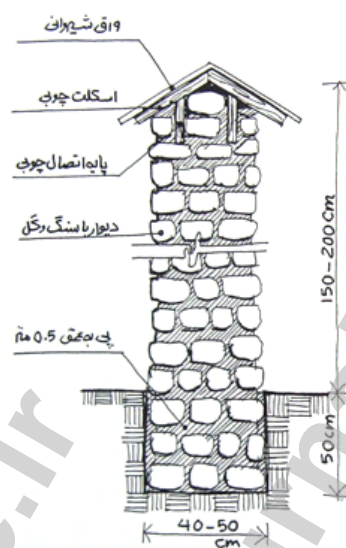
شکل ۸: جزئیات دیوار با سنگ و گل منبع: عمادی، ۱۳۷۷
