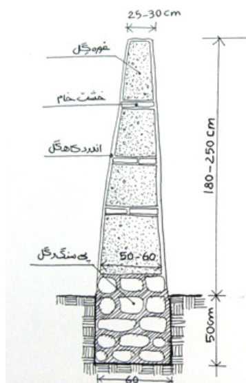
شکل ۹: جزئیات دیوار چینه‌ای منبع: عمادی، ۱۳۷۷
