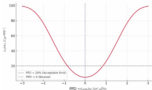
شکل ۶. منحنی نظری PMV-PPD براساس رابطه نمایی استاندارد ASHRAE 55
