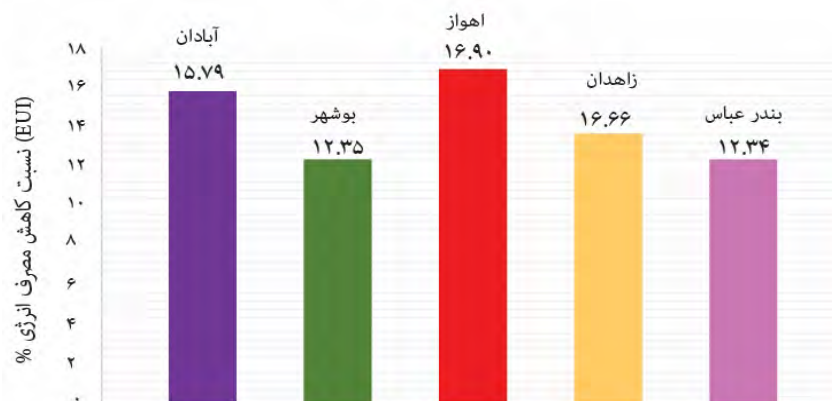
شکل ۹. نمودار شدت کاهش مصرف انرژی در اثر استفاده از جدار ثانویه متحرک در پنج شهر ایران
