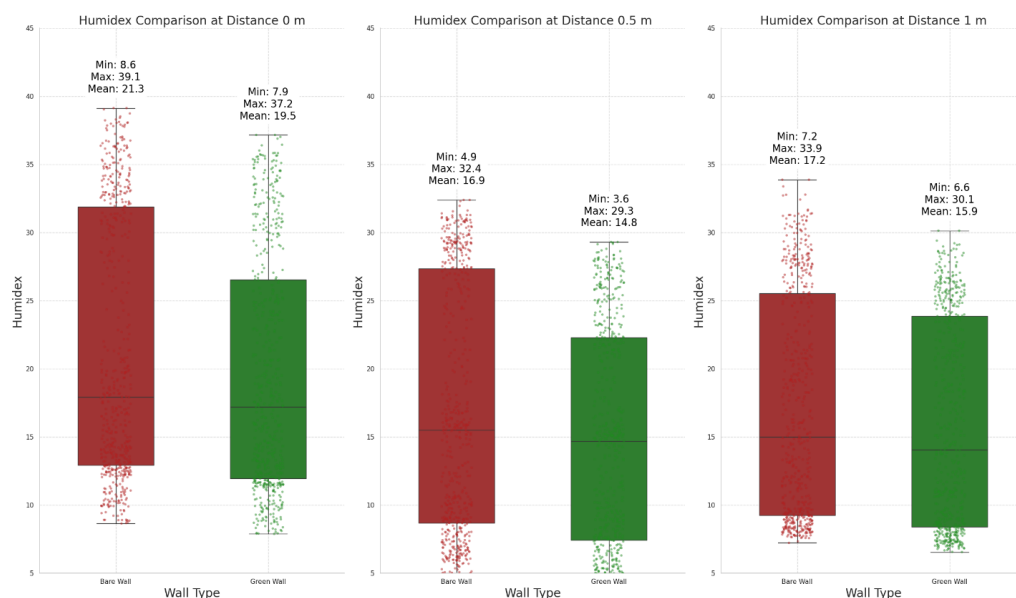
شکل ۶. مقایسه شاخص رطوبت (HD) مجاور دیوار عاری و دیوار سبز در فواصل ۰ متر، ۰٫۵ متر و ۱ متر
