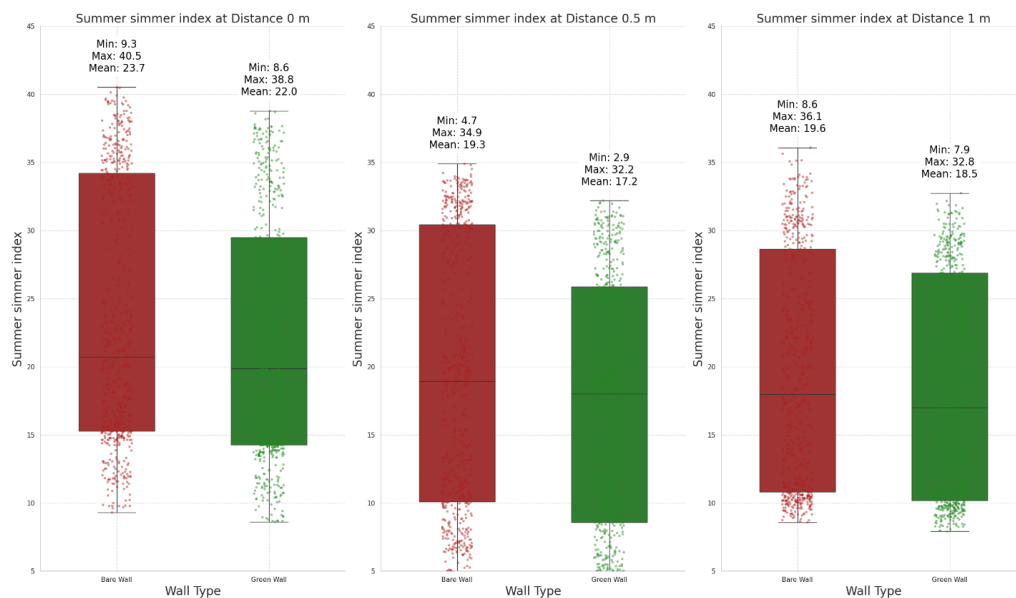
شکل ۸. مقایسه شاخص احساس گرمای تابستانی (SSI) مجاور دیوار عاری و دیوار سبز در فواصل ۰ متر، ۰٫۵ متر و ۱ متر
