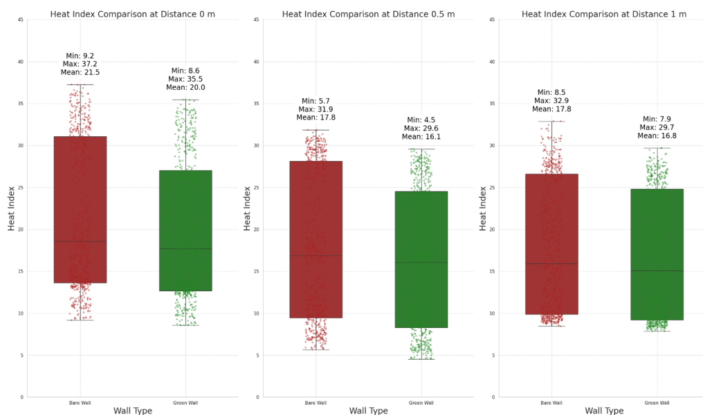
شکل ۵. مقایسه شاخص گرما (HI) مجاور دیوار عاری و دیوار سبز در فواصل ۰ متر، ۰٫۵ متر و ۱ متر
