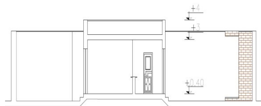
شکل ۲. برش A-A
