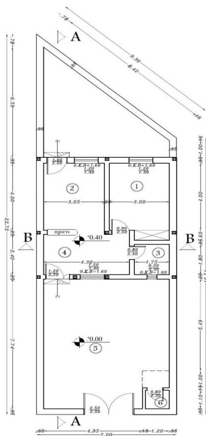
شکل ۱. پلان
