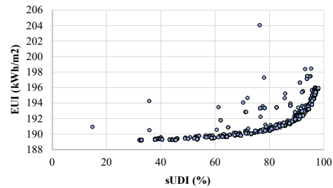
الف) تمامی حالات بررسی شده در بهینه‌سازی در حالت دارای نورگیر جانبی
