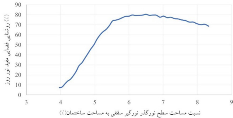
شکل ۲۰. روند تغییر شاخص روشنایی فضایی مفید نور روز با افزایش مساحت نورگیر سقفی
