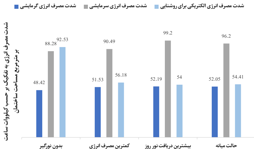
شکل ۱۹. شدت مصرف انرژی به تفکیک انرژی گرمایشی، سرمایشی و روشنایی الکتریکی برای هر یک از سه راه حل بهینه و حالت بدون نورگیر بر حسب کیلووات ساعت بر مترمربع مساحت ساختمان در حالت دارای نورگیر سقفی
