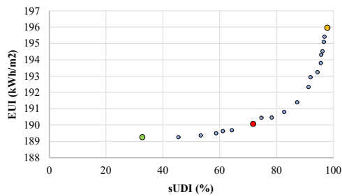
ب) حالات موجود در جبهه پارتو در بهینه‌سازی در حالت دارای نورگیر جانبی
