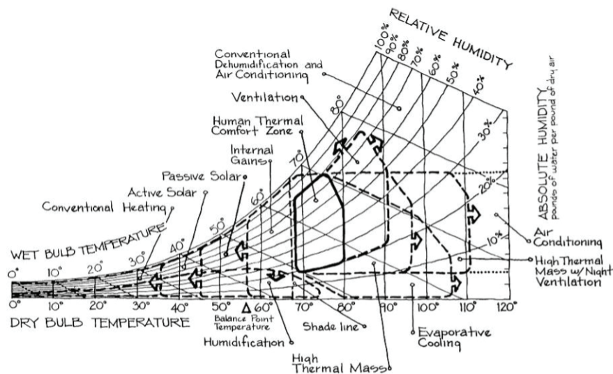
شکل ۱. نمودار زیست‌اقلیمی ساختمانی مایلین-گیونی
